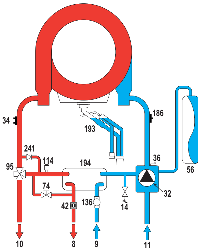
fig. 43- Circuito hidráulico
