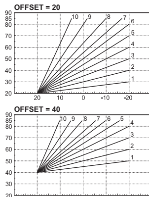
εικ. 15- Παράδειγμα παράλληλης μετατόπισης των καμπυλών αντιστάθμισης
