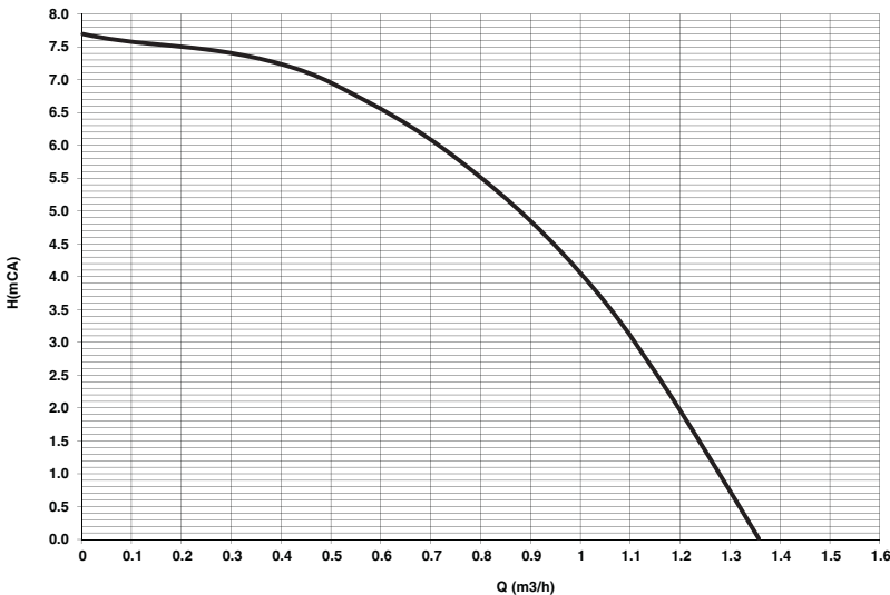
fig. 45- Carga hidrostática residual disponible en la instalación
