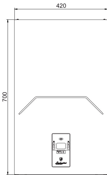
εικ. 38- Μπροστινή όψη
