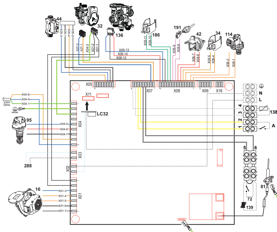
fig. 46- Schemă electrică
