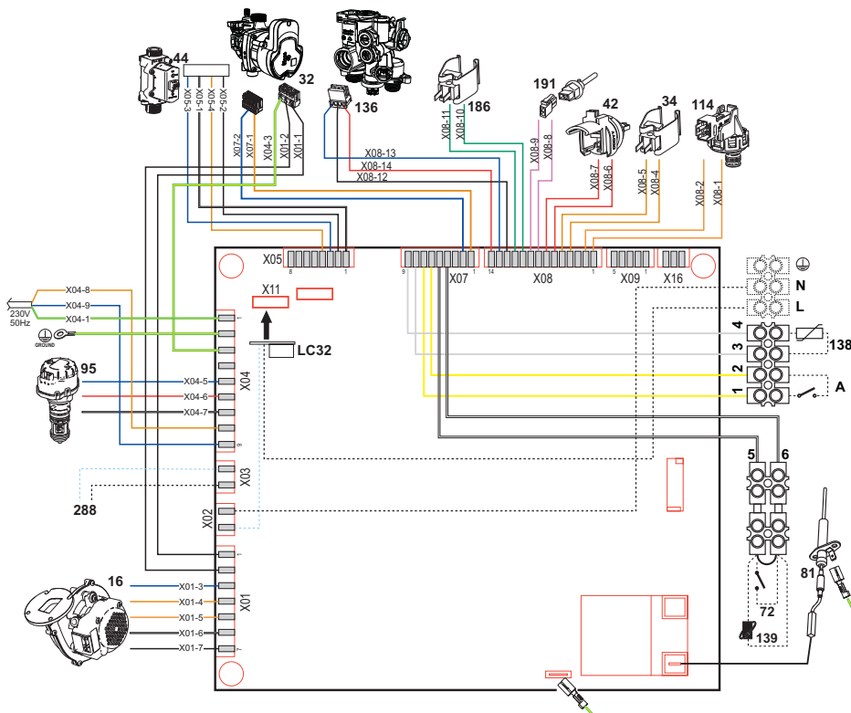
fig. 46 - Schema elettrico
