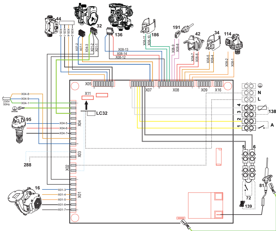
wygląd 46- Schemat elektryczny
