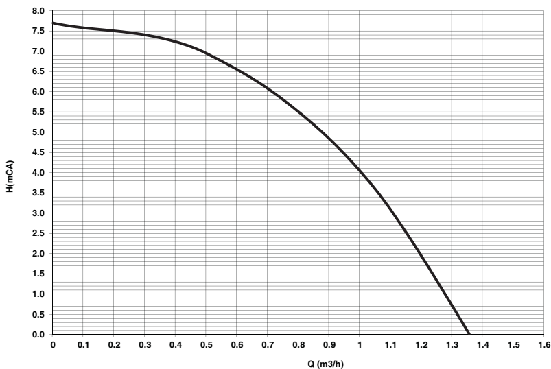
fig. 45- Înălțime de pompare reziduală disponibilă în instalație
