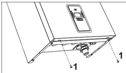
fig. 32- Deschiderea panoului frontal
