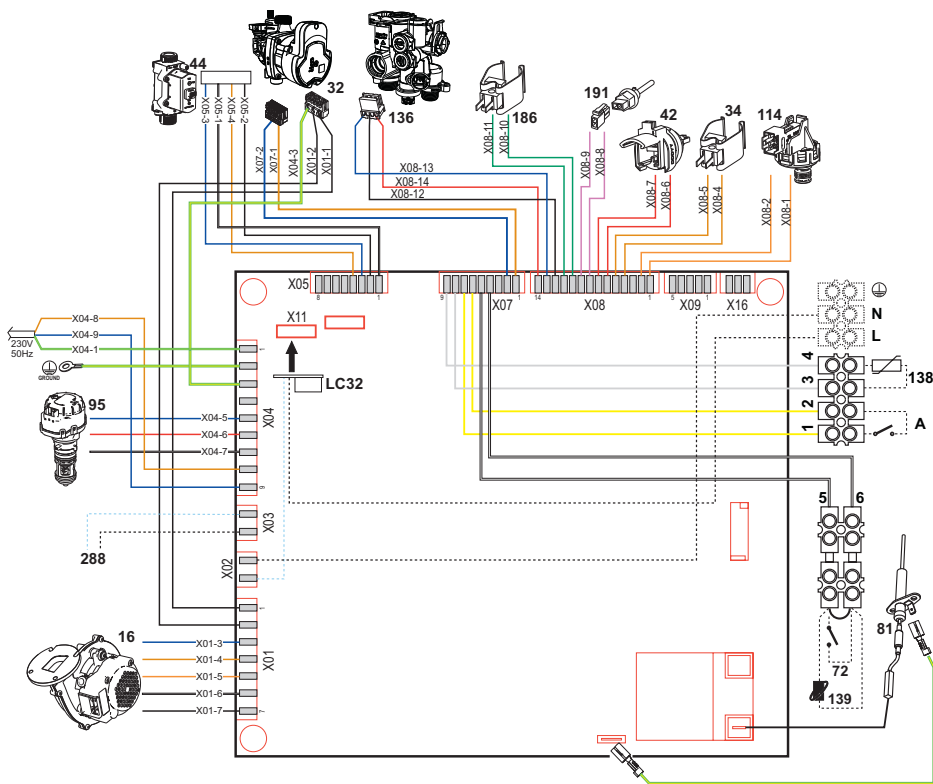
εικ. 46- Ηλεκτρολογικό διάγραμμα
