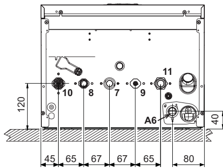
wygląd 41- Widok z dołu
