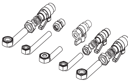
fig. 18 - Kit idraulico
