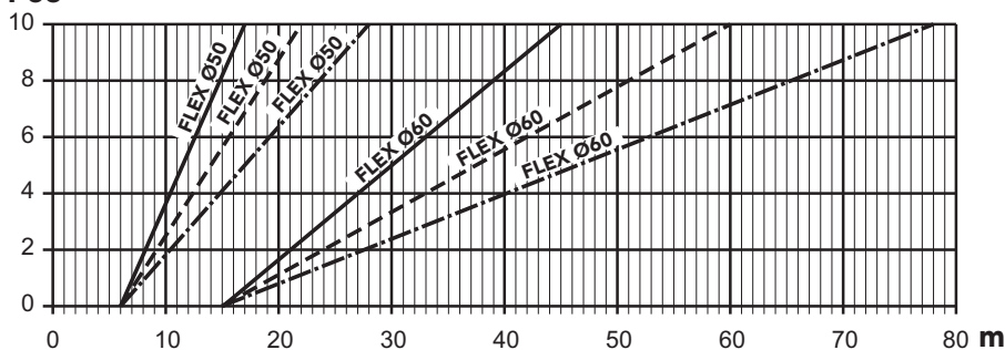
fig. 26- Grafic pentru alegerea parametrului pentru horn
