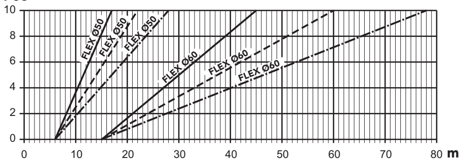
fig. 26 - Grafico per scelta parametro camino
