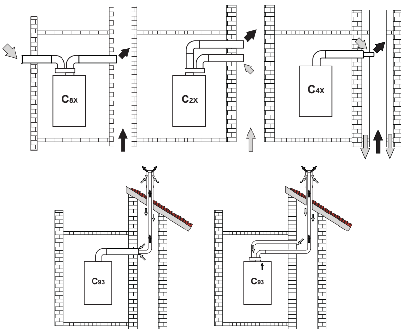
εικ. 27 Παραδείγματα σύνδεσης σε καπνοδόχους (⇒ = Αέρας / ⇒ = Κουσαέρια)
