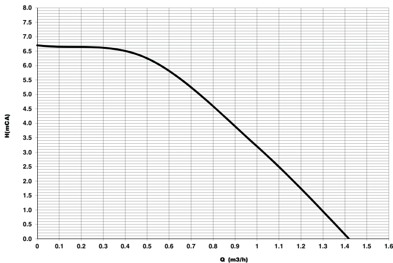
εικ. 44- Διαθέσιμο υπολειπόμενο μανομετρικό ύψος στην εγκατάσταση
