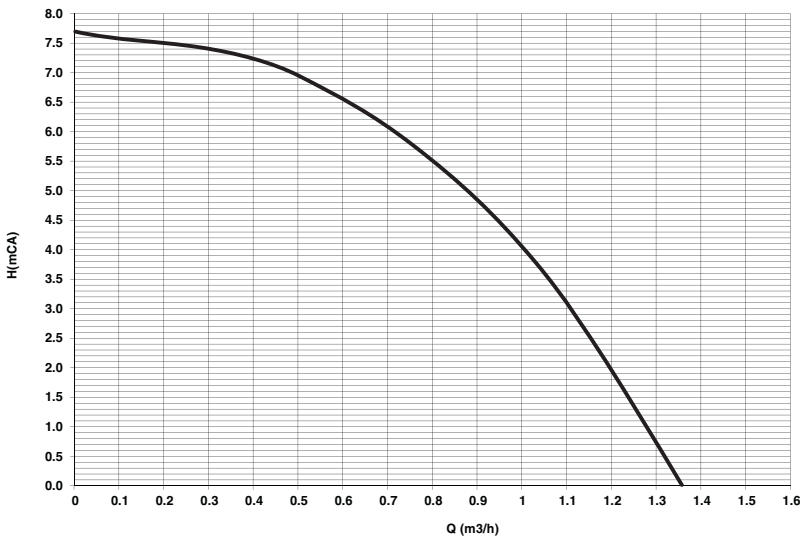
wygląd 45- Wysokość podnoszenia dostępna w instalacji
