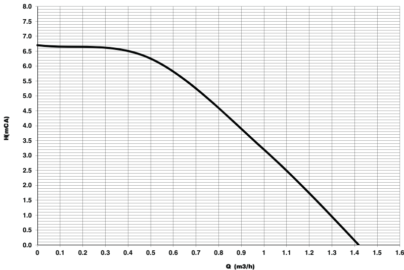
fig. 44- Carga hidrostática residual disponible en la instalación
