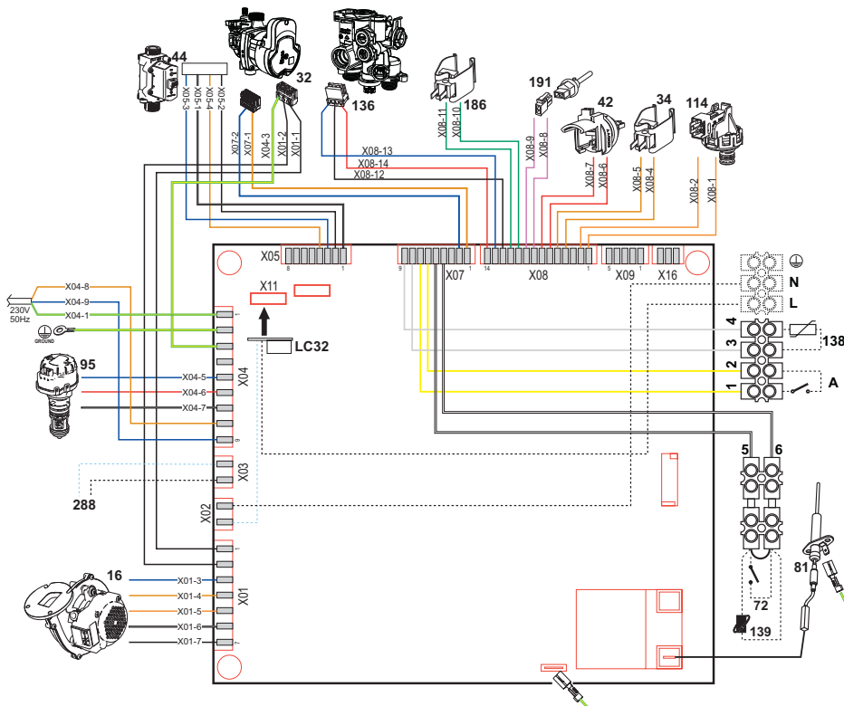
fig. 46- Wiring diagram
