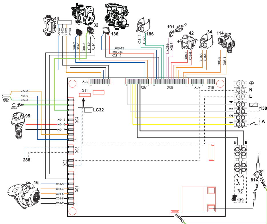
fig. 46- Esquema eléctrico
