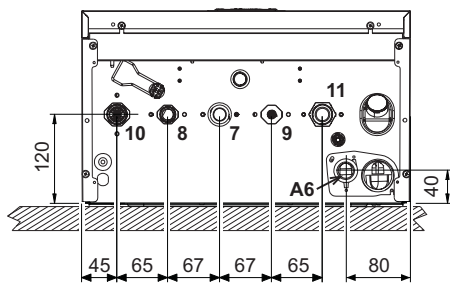
fig. 37- Vedere de jos
