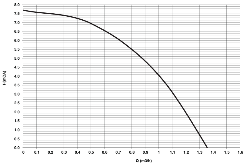
εικ. 45- Διαθέσιμο υπολειπόμενο μανομετρικό ύψος στην εγκατάσταση
