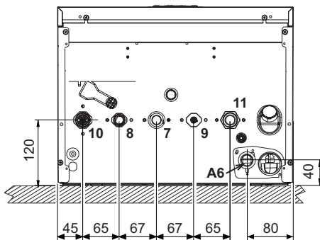
fig. 41 - Vista dal basso
