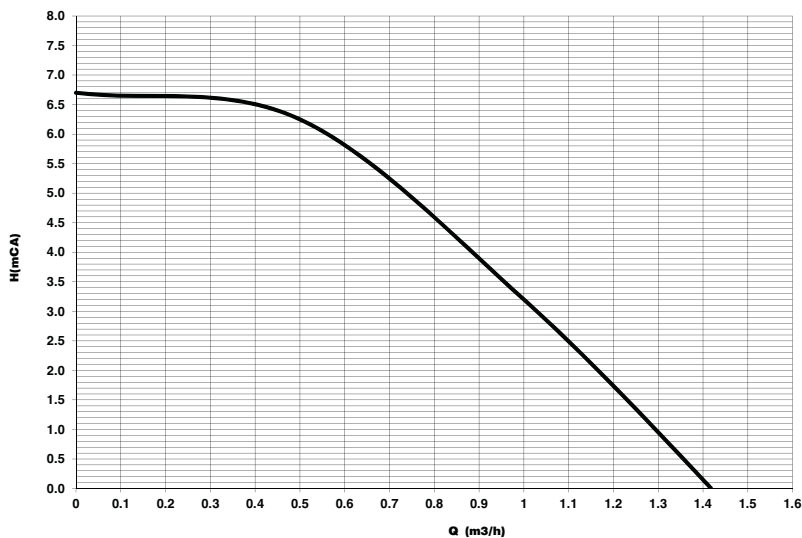
fig. 44- Înălțime de pompare reziduală disponibilă în instalație
