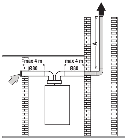
εικ. 25- Διάγραμμα μόνο για τοποθέτηση εύκαμπτου σωλήνα
